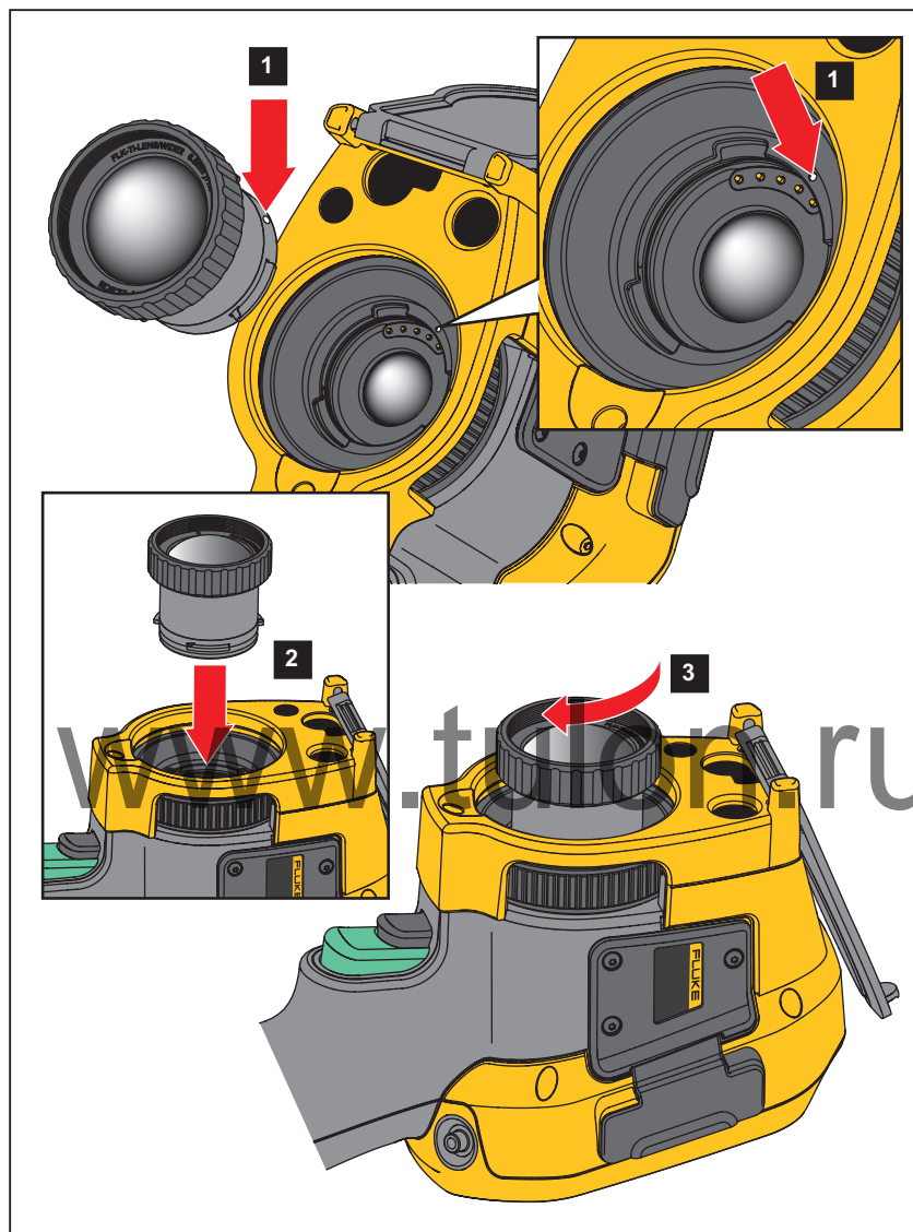
Рисунок 1. Установка дополнительного объектива
