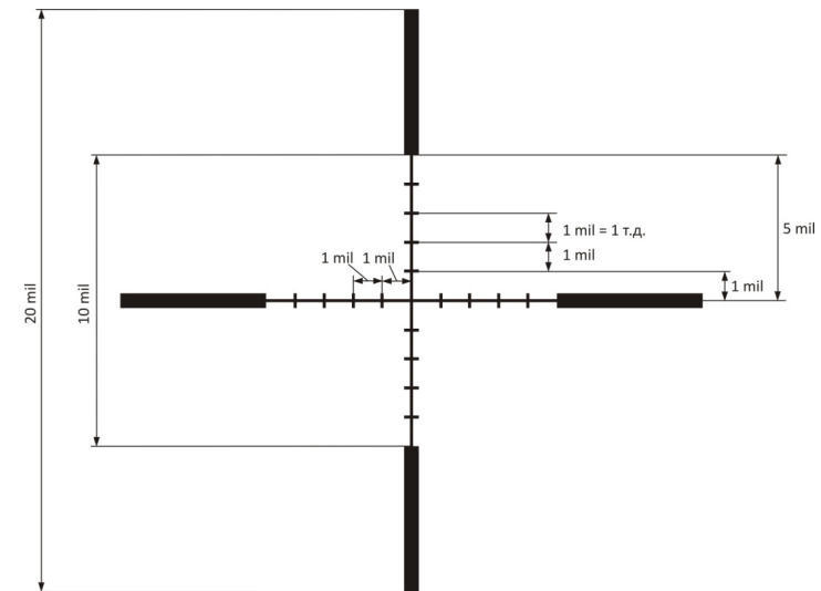
Рисунок 31 – Прицельная сетка (размер в миллирадианах
