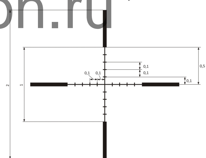
Рисунок 32 – Прицельная сетка (размер в м/100м дистанции)
