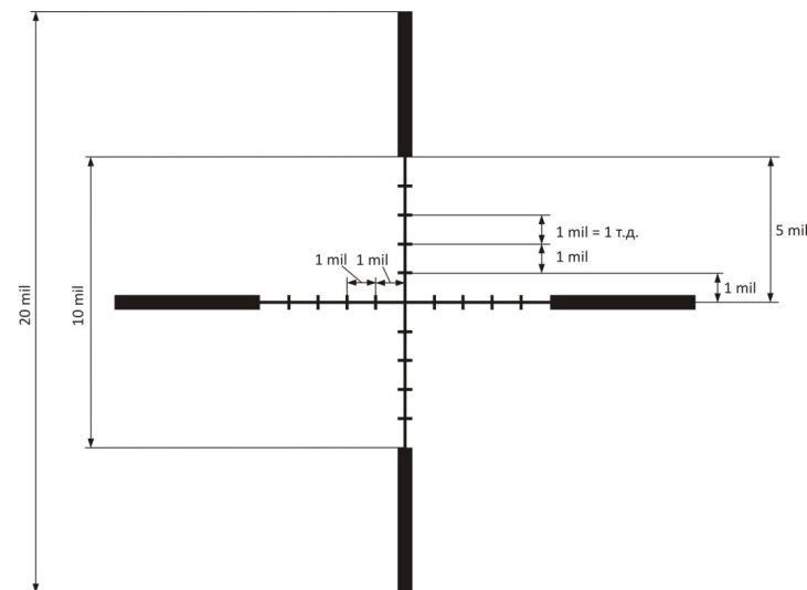
Рисунок 31 – Прицельная сетка (размер в миллирадианах
