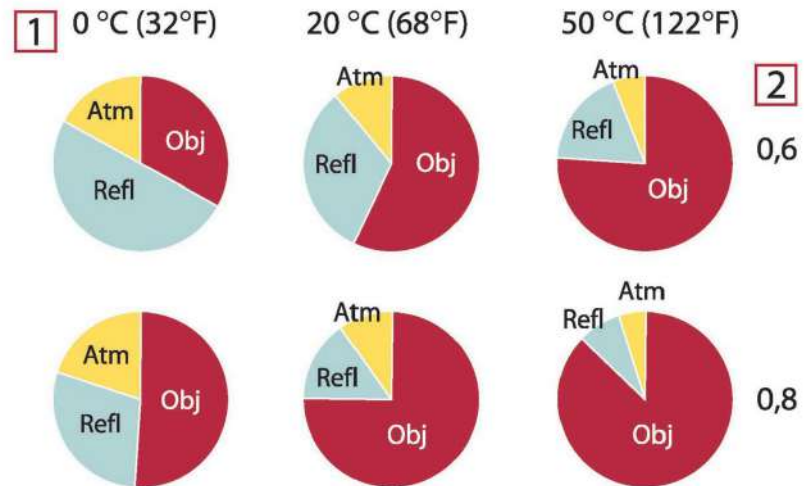
Figure 40.2 Относительные величины источников излучения при различных условиях измерений (SW-камера). 1: Температура объекта; 2: Светимость; Obj: Излучение объекта; Refl: Отраженное излучение; Atm: излучение атмосферы. Фиксированные параметры: \tau = 0,88 ; T_{refl} = 20^\circ\text{C} ; T_{atm} = 20^\circ\text{C} .
