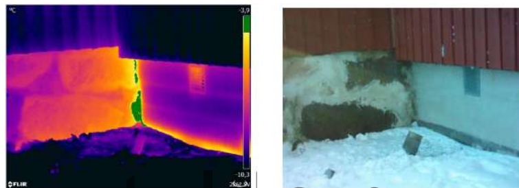
Figure 36.10 Фундаментная стена: соединение между старой (слева на изображении) и новой (справа на изображении) частями здания. Изотерма выделяет зону утечки воздуха.
