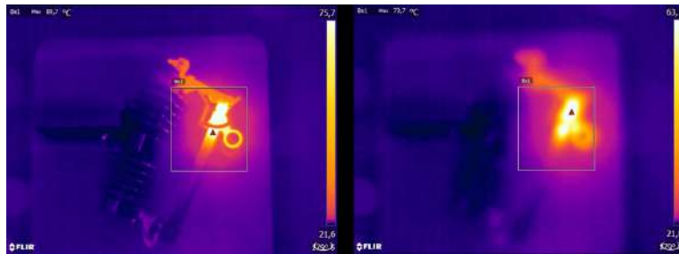
Figure 36.2 Сфокусированное тепловизионное изображение (левое) с максимальной температурой T_{\text{макс.}} = 89,7^{\circ}\text{C} и нефокусированное тепловизионное изображение (правое) с максимальной температурой T_{\text{макс.}} = 73,7^{\circ}\text{C} .
