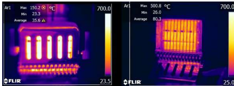
Figure 36.5 Изображение того же объекта, снятое при разных диапазонах температур: от -20 до 120^{\circ}\text{C} (левое изображение) и от 0 до 650^{\circ}\text{C} (правое изображение). Температура на левом изображении выводится с предупреждающим знаком (красный круг с белым крестом), так как измеренные значения находятся за пределами откалиброванного диапазона.
