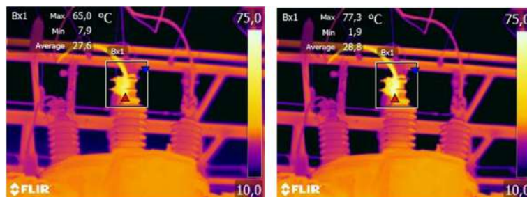
Figure 36.11 Изменение коэффициента излучения для сохраненного изображения. Максимальная температура составляет 65,0°C для \epsilon = 0,95 на левом изображении и 77,3°C для \epsilon = 0,7 на правом изображении.
