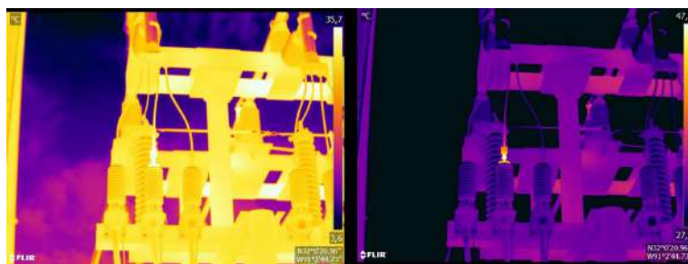
Figure 36.8 Тепловизионное изображение в автоматическом режиме (левое изображение) и в ручном режиме (правое изображение). Отрегулированный интервал температур увеличивает контрастность изображения и делает неисправности более наглядными.
