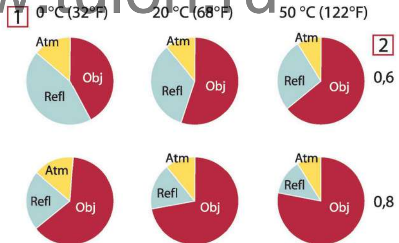
Figure 40.3 Относительные величины источников излучения при различных условиях измерений (LW-камера). 1: Температура объекта; 2: Светимость; Obj: Излучение объекта; Refl: Отраженное излучение; Atm: излучение атмосферы. Фиксированные параметры: \tau = 0,88 ; T_{refl} = 20^\circ\text{C} ; T_{atm} = 20^\circ\text{C} .
