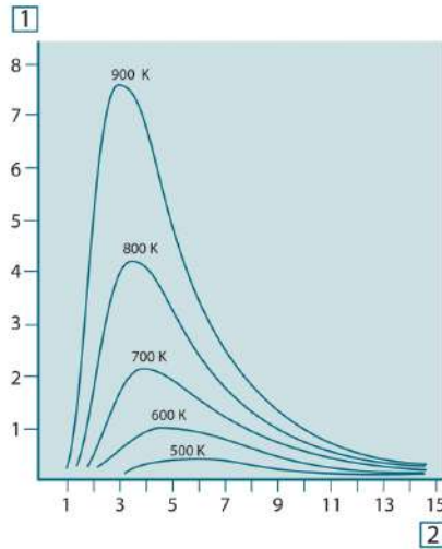
Figure 39.4 Кривые спектральной излучательной способности черного тела в соответствии с законом Планка, построенные для разных значений абсолютной температуры 1: Спектральная излучательная способность ( \text{Вт/см}^2 \times 10^3(\text{мкм}) ); 2: Длина волны (мкм).
