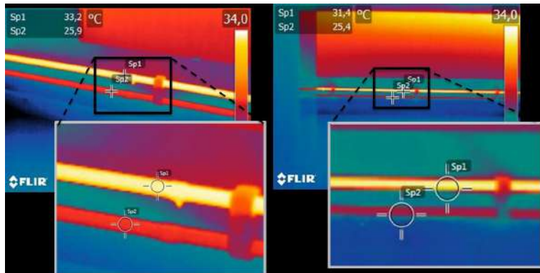
Figure 36.7 Подводящие и отводящие трубопроводы радиаторов в офисном помещении с открытой планировкой. Левое изображение было снято с расстояния 1 метр: измерительная точка заполнена, измерение температуры правильное. Правое изображение было снято с расстояния 3 метра: измерительная точка не полностью заполнена, измеренные значения температуры неправильные (31,4 и 24,4°C вместо 33,2 и 25,9°C).
