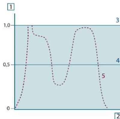
Figure 39.9 Спектральный коэффициент излучения трех типов излучателей 1: Спектральный коэффициент излучения; 2: Длина волны; 3: Черное тело; 4: Серое тело; 5: Избирательный излучатель.
