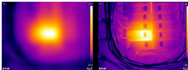
Figure 36.1 На нефокусированном изображении (левое) видны только неясные «мазки теплоты». На сфокусированном изображении (правое) четко показан наблюдаемый объект и теплые места объекта.
