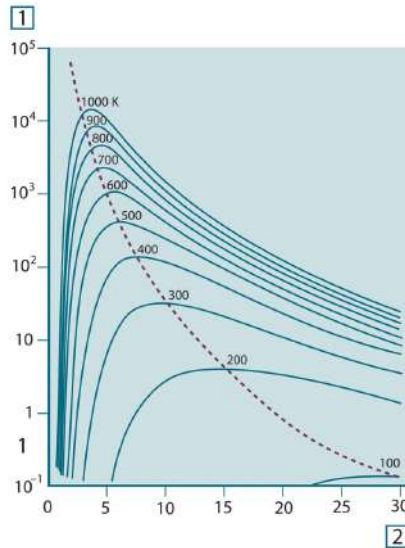
Figure 39.6 Кривые Планка, построенные в полулогарифмическом масштабе от 100 К до 1000 К. Пунктирная линия представляет геометрическое место точек максимума излучательной способности при каждой температуре согласно закону смещения Вина 1: Спектральная излучательная способность ( W/cm^2 \cdot \mu m ); 2: Длина волны ( \mu m ).
