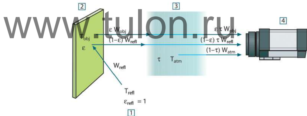
Figure 40.1 Схематическое представление ситуации при общих термографических измерениях: 1: Среда; 2: Объект; 3: Атмосфера; 4: Камера
