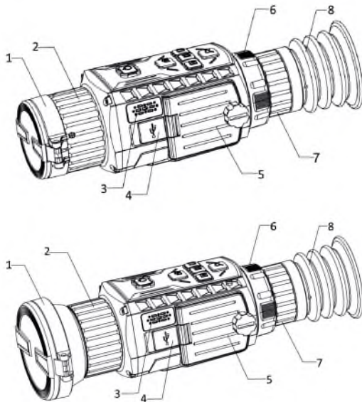
Рис. 1-1 Основные части двух типов тепловизионных прицелов
