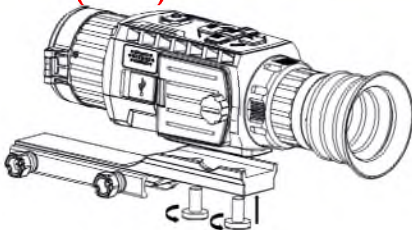
Рис. 2-5. Установка устройства и затягивание винтов
