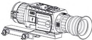
Рис. 2-6. Закрепление устройства
