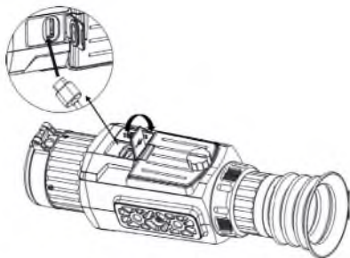
Рис. 2-1. Подключение кабелей
