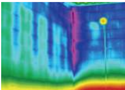
Рис. 5-24. Тепловой рисунок блочной стены показывает проникновение влаги в месте соединения двух стен, а так же неоднородности строительных конструкций.
