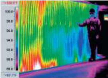
Рис. 5-42. Теплые участки на поверхности котла могут быть вызваны износом огнеупорной футеровки, течь воздуха или обеими причинами.
