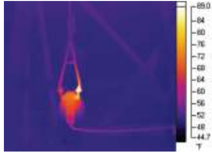
Рис. 5-37. Поскольку параллельные пути для прохождения тока существуют во многих разъединителях, перегрев может показывать нормальное соединение, а местом, где на самом деле существует проблема, может быть холодная часть.
