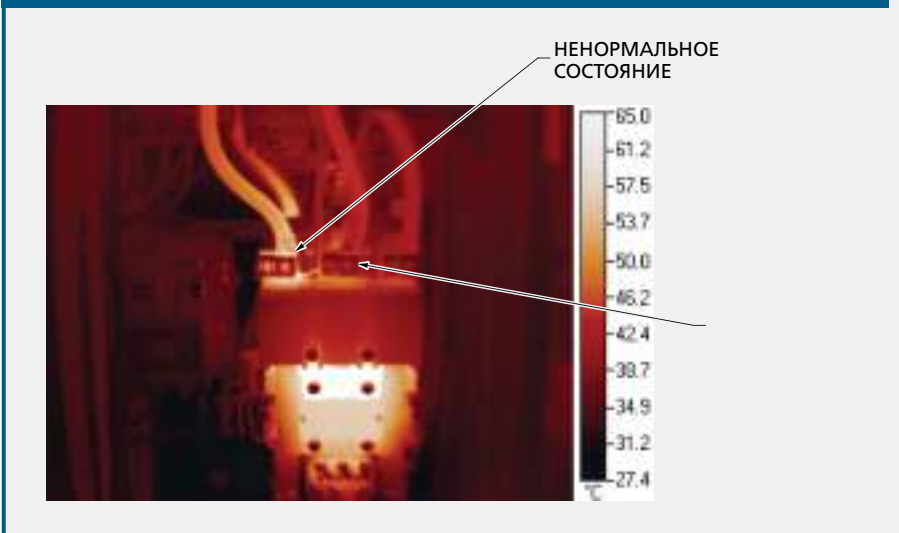
Рис. 2-1. Тепловые сигнатуры работающего оборудования могут быстро указать на нормальное и ненормальное состояние.
