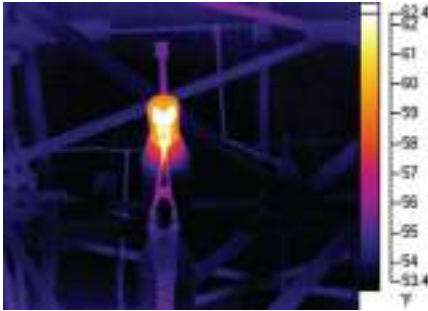
Рис. 5-36. Ненормально высокое сопротивление вызывающее нагрев разъединителя часто представляет серьезную дорогостоящую проблему, поскольку даже сравнительно невысокие температуры могут вызвать повреждения.
