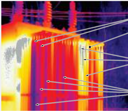
Рис. 4-2. Естественная конвекция наблюдается, когда теплое масло поднимается вверх, а холодное опускается вниз, как происходит в охлаждающих трубках маслонеполненного трансформатора.
