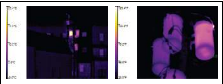
Рис. 5-35. Некоторые проблемы можно обнаружить даже на большом расстоянии (слева) с помощью тепловизора. Более тщательный анализ часто требует использования телескопического объектива или подойти ближе (справа) к оборудованию.
