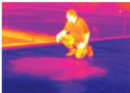
Рис. 5-53. Область с влажной теплоизоляцией крыши проявляется в виде теплого участка на крыше ранним вечером, когда условия самые подходящие для тепловизионной съемки.
