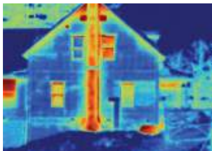
Рис. 5-48. Тепловое изображение наружного вида здания может четко указать на проблемные зоны, такие как светлые участки, где отсутствует теплоизоляция.
