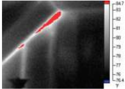
Рис. 5-43. Красный цвет насыщения цветовой палитры четко указывает плохую укладку теплоизоляции из стекловолкна в наклонной кровле.
