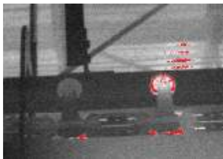
Рис. 5-52. Ненормальный нагрев подшипника конвейерной ленты может привести к чрезмерному расходу энергии и со временем к растяжению цепи.
